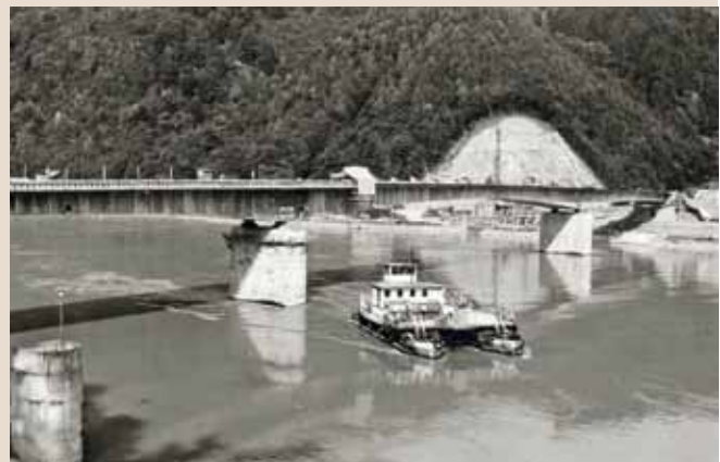
Foto: Die Donaubrücke Ardagger-Grein wurde 1967 nach dreijähriger Bauzeit eröffnet. Davor konnte man die Donau mit einer Rolfähre, wie am Foto ersichtlich, überqueren. © zVg
