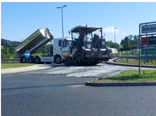
Die Fertigungsmaschine bei den Asphaltierungsarbeiten am Kreisverkehr Schnalle.
