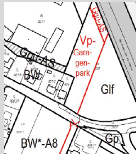
Auszug aus dem Flächenwidmungsplan.
