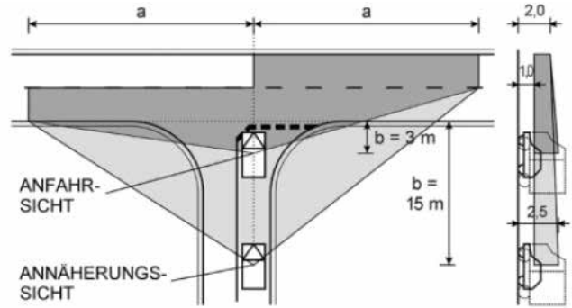
Abbildung 29: Schemaskizze eines Sichtraumes im Knoten
