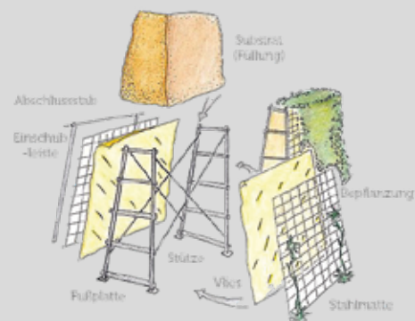
Aufbau des begrünten Lärmschutzes.
