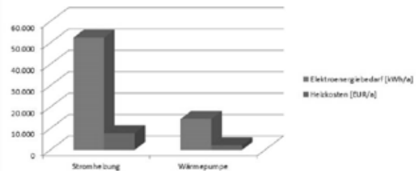
Deutlich zu erkennen ist die Ersparnis an Primärenergie und Heizkosten mit der Wärmepumpenlösung.
